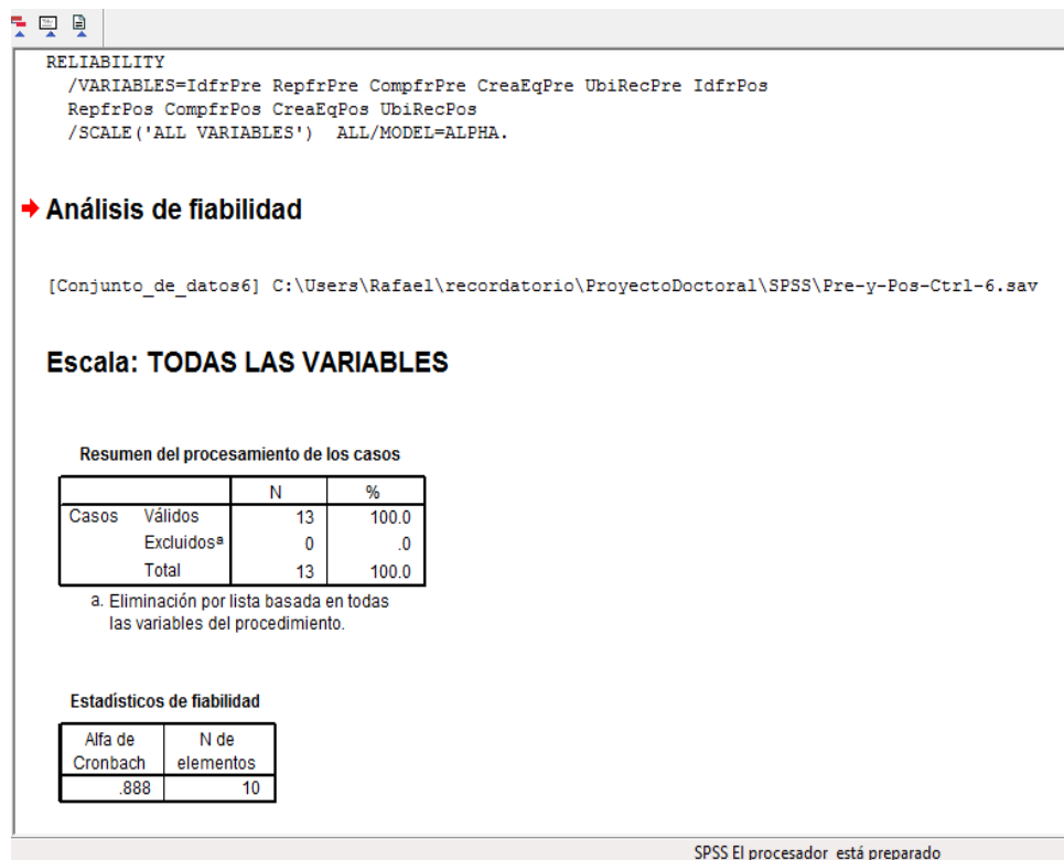
Fig. No. 4.33 Prueba de fiabilidad alfa de Cronbach – Grupo control sexto grado. Fuente: Elaboración propia (2014). Procesamiento estadístico de datos con el programa SPSS ver. 15.0 para Windows .
