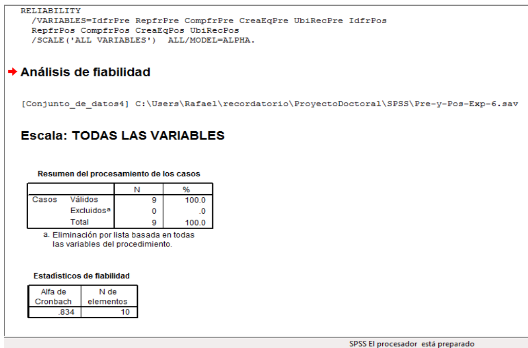
Fig. No. 4.34 Prueba de fiabilidad alfa de Cronbach – Grupo experimental sexto grado. Fuente: Elaboración propia (2014). Procesamiento estadístico de datos con el programa SPSS ver. 15.0 para Windows .
