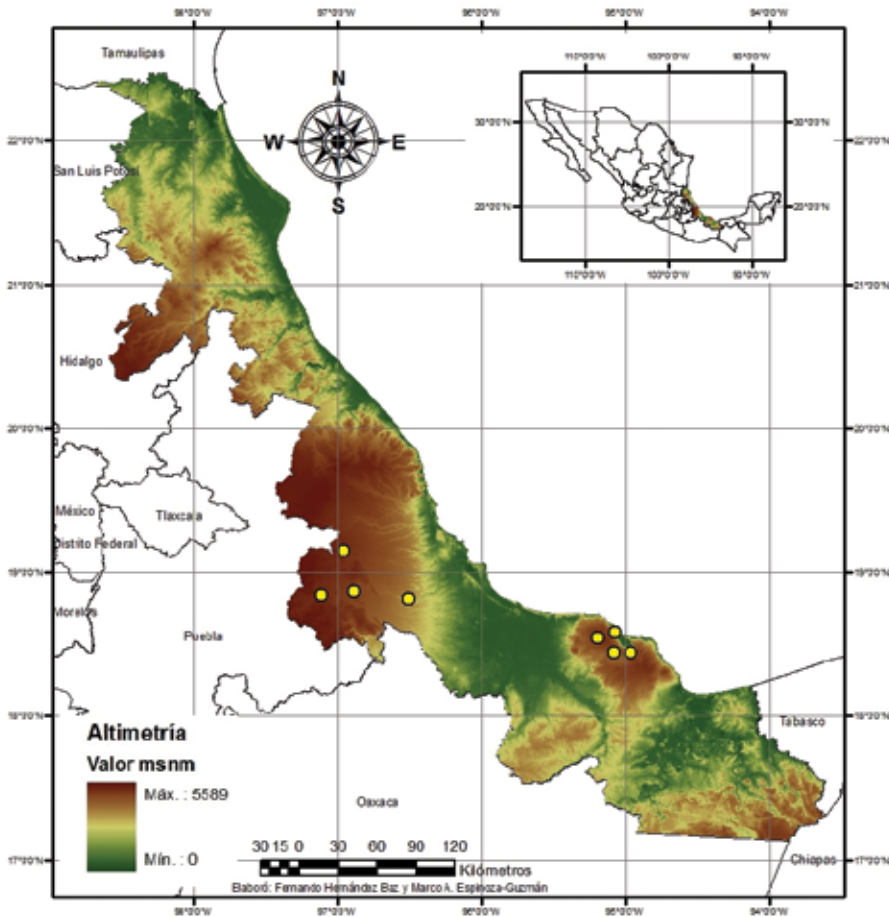
Figura 2. Distribución en Veracruz de Morpho polyphemus luna Butler, 1869. Los puntos amarillos sindicán su distribución conocida. Fuente: Vargas-Fernández et al. , 2008; Hernández-Baz et al. , 2010; Luis-Martínez, 2011.
