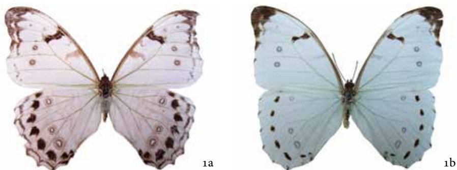
Figura 1a. Vista dorsal macho y 1b, vista dorsal hembra de Morpho polyphemus luna Butler, 1869 fotos: F. Hernández-Baz.
