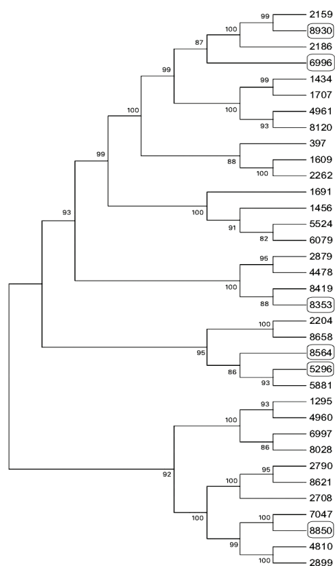
Figura 4. Reconstrucción filogenética de agrupamiento jerárquico aglomerado simple (UPGMA) (Sneath y Sokal, 1973) de secuencias de nucleótidos identificadas en parte del genoma de M. roleri CPMRT01. Se muestra el árbol óptimo con la suma de la longitud de rama = 0.00725912. El porcentaje de árboles replicados en los taxones asociados, agrupados en la prueba de arranque (500 repeticiones) se muestran junto a las ramas. Cada número (etiqueta) corresponde al cóntigo identificado. Los cóntigos predichos se encuentran en recuadros.
