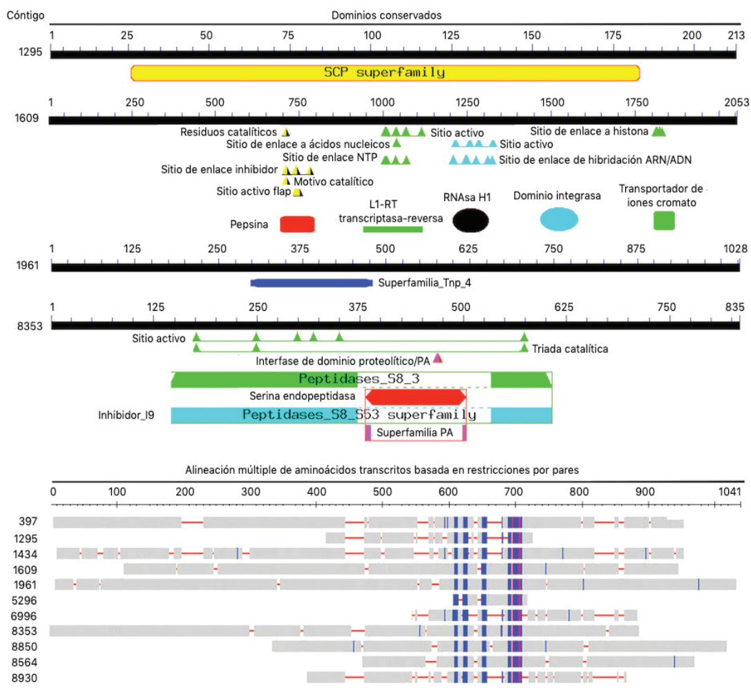
Figura 5. Representación gráfica de la predicción de dominios conservados hipotéticos con máximas similitudes identificados en parte del genoma de M. roseri CPMRT01. La alineación inferior múltiple de aminoácidos basada en restricciones por pares muestra 11 transcritos que sugieren similitud con sus secuencias residuales en donde el color azul representa regiones similares y el rojo regiones altamente conservadas.
