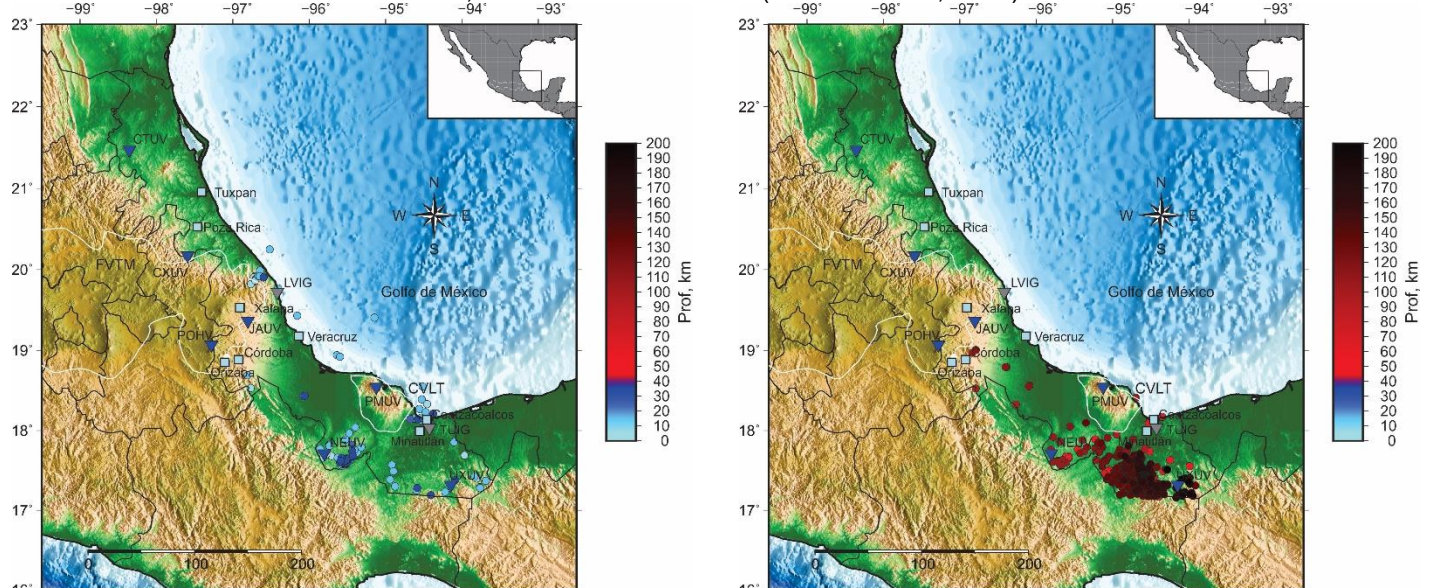
Figura 2. Mapa de sismicidad cortical (izquierda) y la sismicidad intraplaca (derecha) en el estado Veracruz reportada por el SSN para el periodo comprendido del 1 de enero al 31 de diciembre de 2021.
