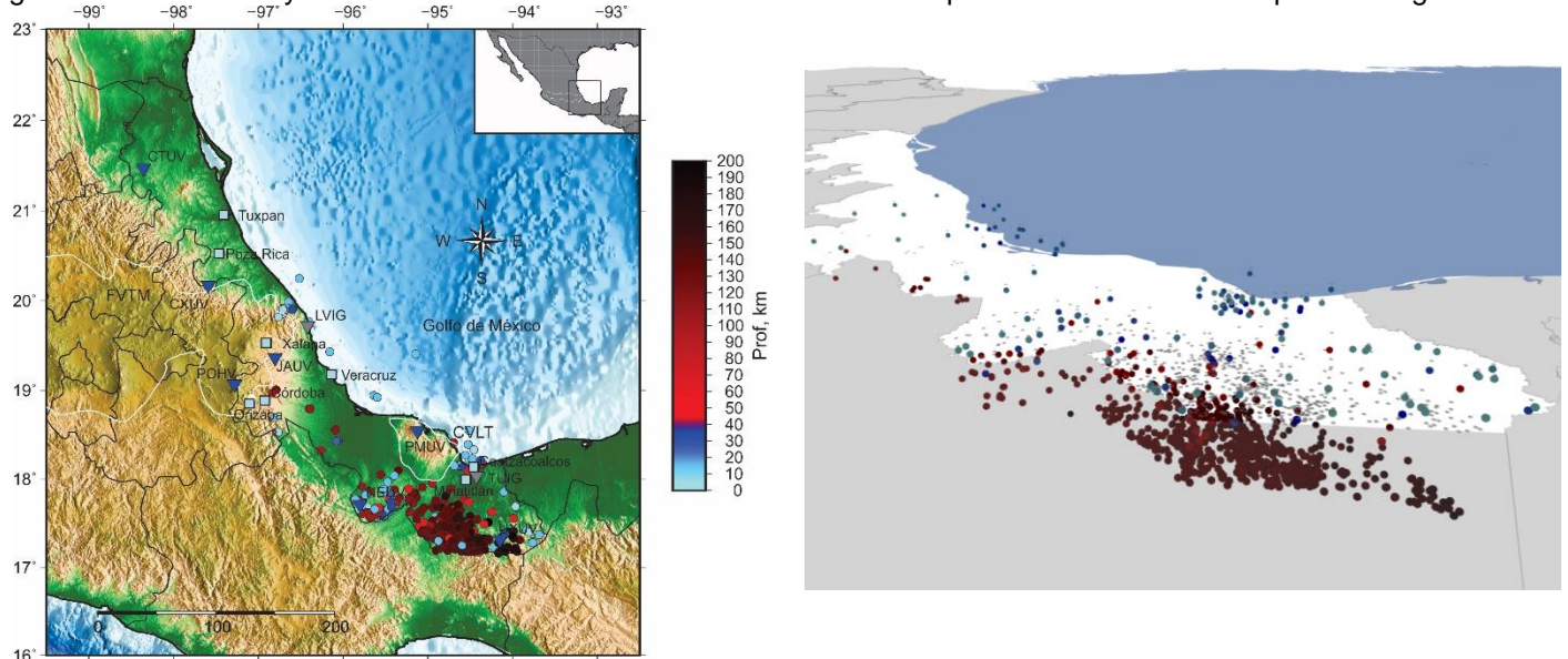
Figura 1. Mapa de sismicidad general en Veracruz reportada por el SSN para el periodo comprendido del 1 de julio al 31 de diciembre de 2021. (a) Vista en planta. (b) Representación en 3-D. Los círculos azules representan a los sismos ocurridos en la corteza continental, en tanto que los rojos corresponden a los localizados en la corteza oceánica. Los triángulos invertidos en color azul y gris señalan la ubicación de las estaciones de la Red Sísmica de Banda de Veracruz (RSBAV, Córdoba et al. , 2018) y las del SSN respectivamente en el estado de Veracruz. Los cuadrados en azul, señalan la localización de las principales ciudades de la entidad veracruzana.
