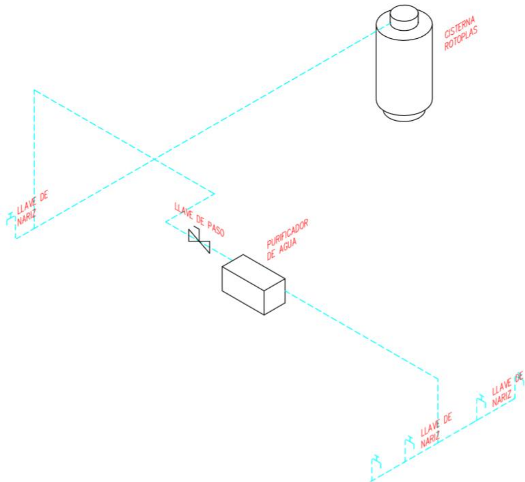
Isométrico, Instalación de sistema de purificación de agua en la Facultad de Contaduría y Administración, Ixtaczoquitlán.
