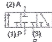
Válvula 3/3 vías, posición central cerrada
