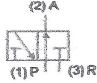
Válvula 3/2 vías Normalmente Cerrada
