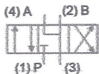
Válvula 4/3 vías, posición central, con conductos de trabajo a escape
