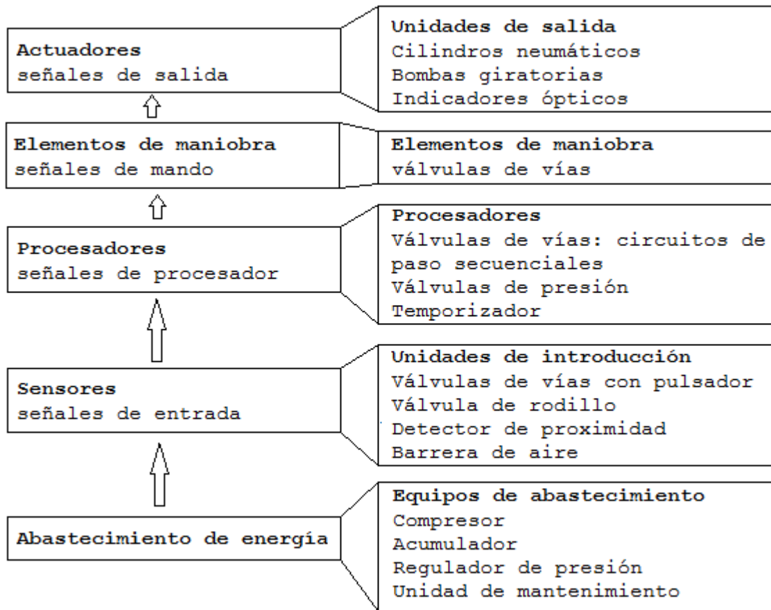
Ilustración 1 Esquema de mando neumático
