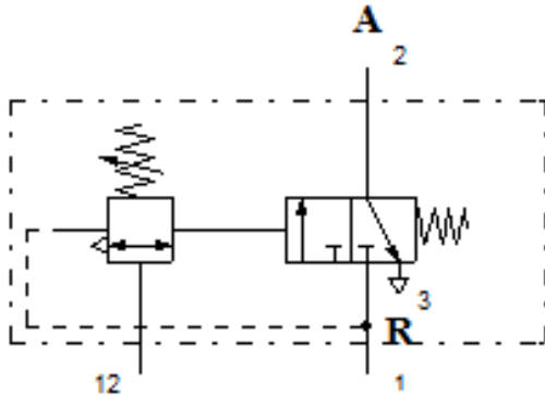
Válvula de secuencia normalmente cerrada
