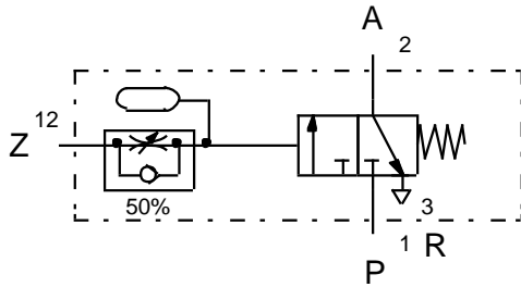
Temporizador Normalmente cerrado
