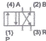
Válvula 4/2 vías
