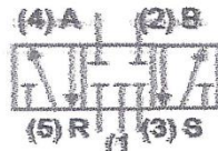
Válvula 5/3 vías, posición central cerrada
