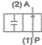
Válvula 2/2 vías Normalmente Abierta
