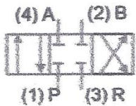
Válvula 4/3 vías, posición central cerrada
