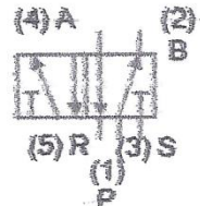
Válvula 5/2 vías
