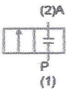
Válvula 2/2 vías Normalmente Cerrada
