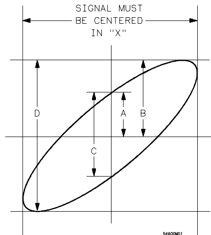
Phase shift Parameters
