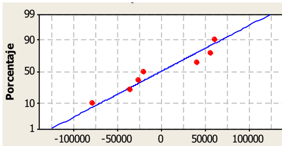
Figura 6. Gráfica de probabilidad normal de los residuos del modelo.
