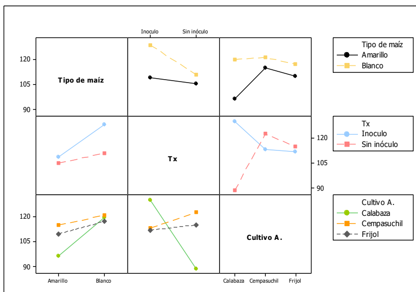
Figura 2. Gráfico de interacciones entre factores para el peso de la mazorca.
