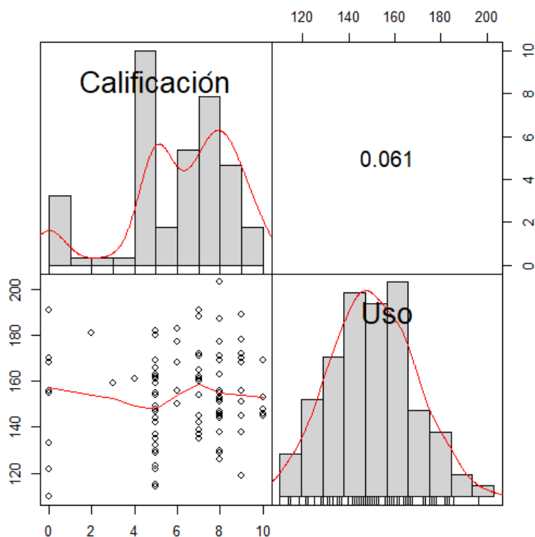
Figura 1. Matriz de correlación entre la calificación y el uso del teléfono inteligente.
