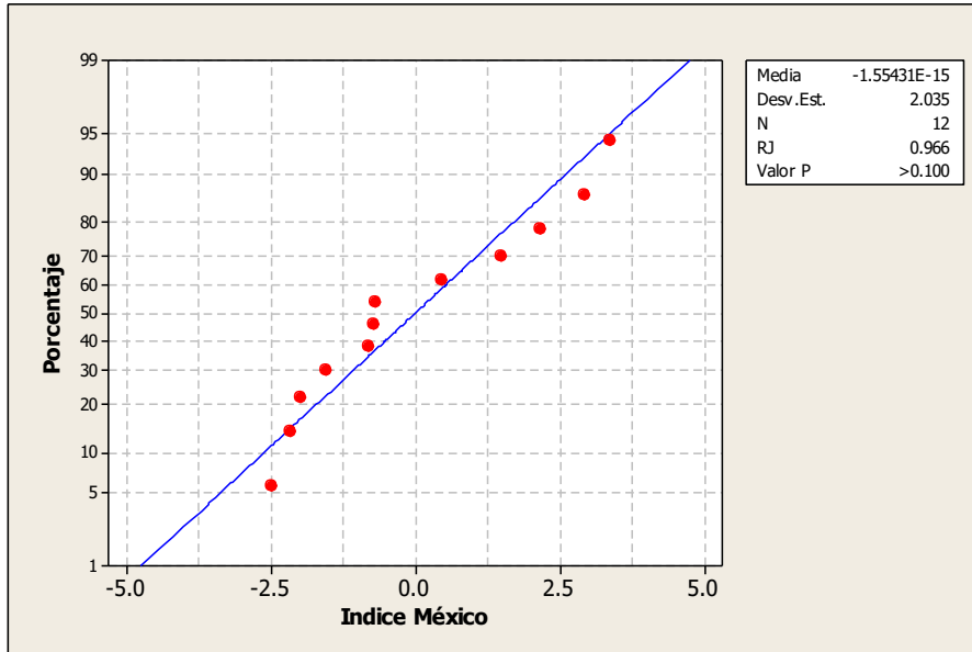
Figura 12. Gráfica de la probabilidad normal del Índice Sector Cultural México.
