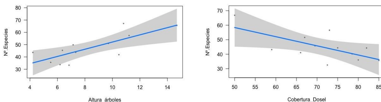
Figura 4. Regresiones parciales para la predicción del número de especies de hormigas en función de la altura de los árboles y la cobertura del dosel en 12 sitios de estudio.
