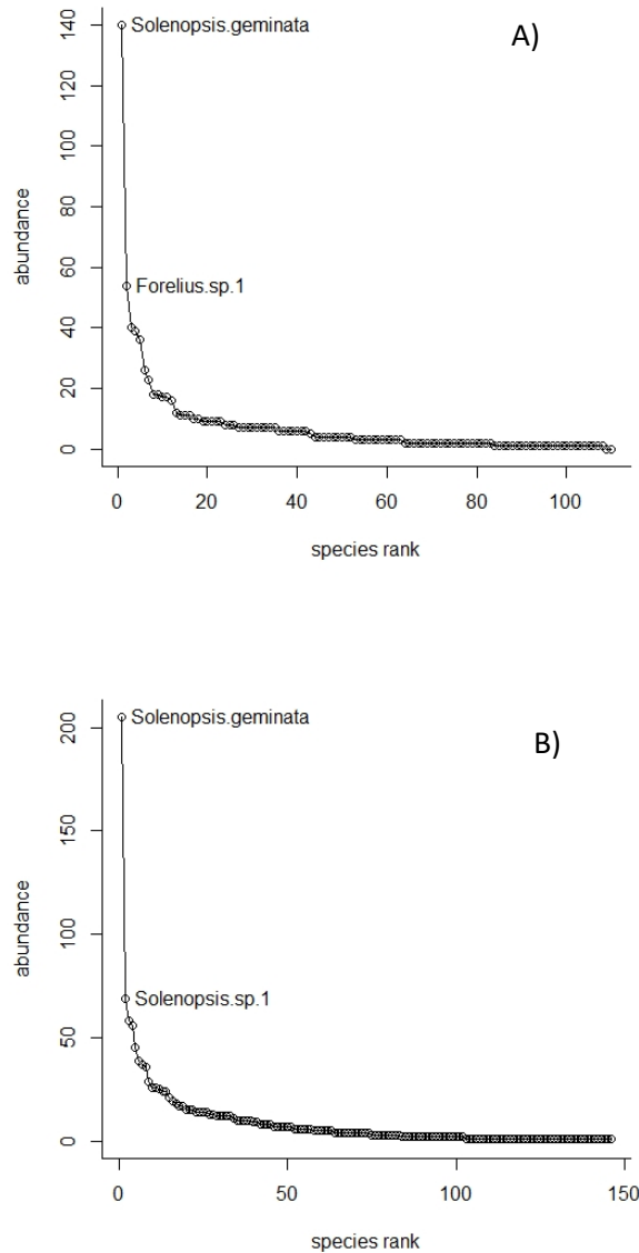
Figura 3. Curva de abundancias de especies de hormigas, A) grupo de fincas con estructura arbórea baja, B) grupo de fincas con estructura arbórea alta.
