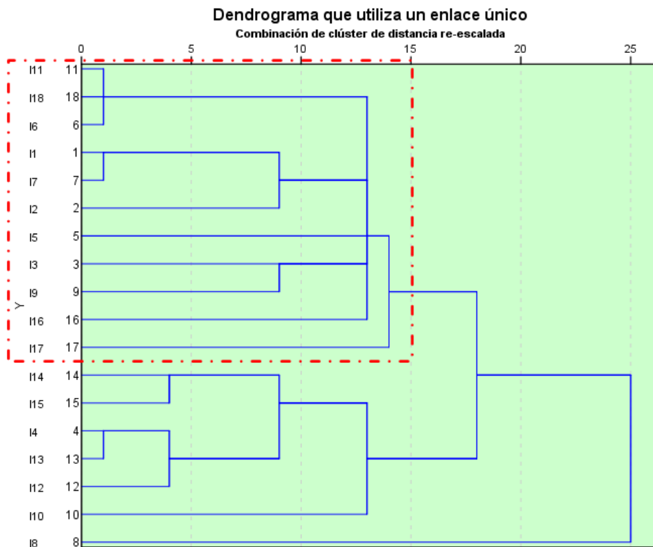
Figura 5. Dendrograma correspondiente a la agrupación de alumnos con nivel de aprovechamiento destacado.
