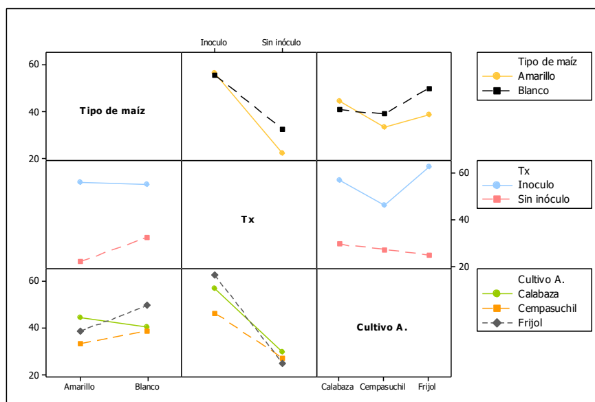
Figura 3. Gráfico de interacciones entre factores para el porcentaje de colonización
