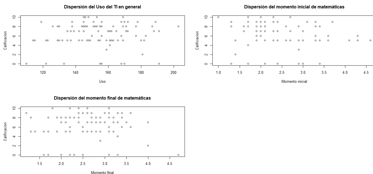
Figura 2. Diagramas de dispersión.
