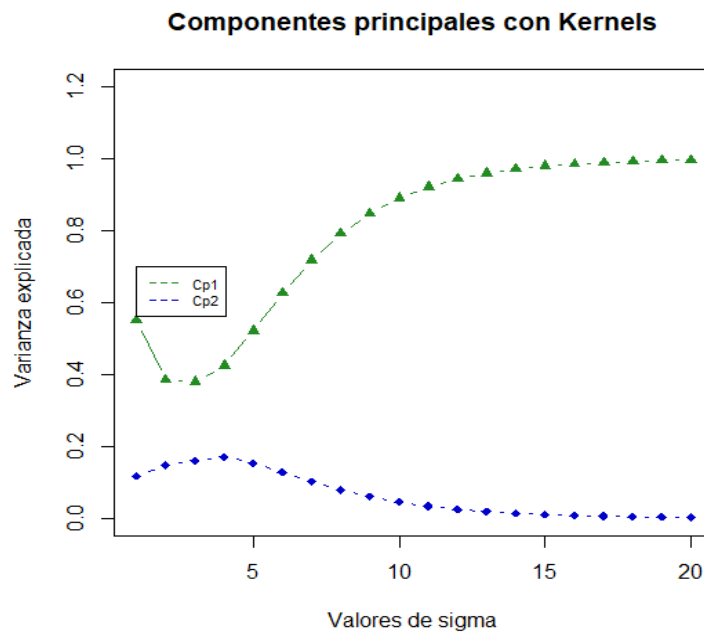
Figura 3. Comportamiento de la varianza explicada por valor del parámetro sigma para el año 2020.
