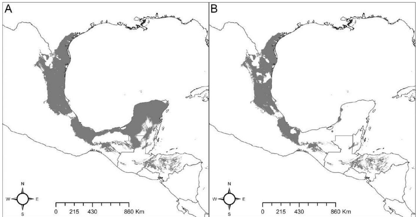
Figura 1. A. Área potencial de distribución (presente). B. Área de distribución prevista en un escenario de cambio climático (2070).
