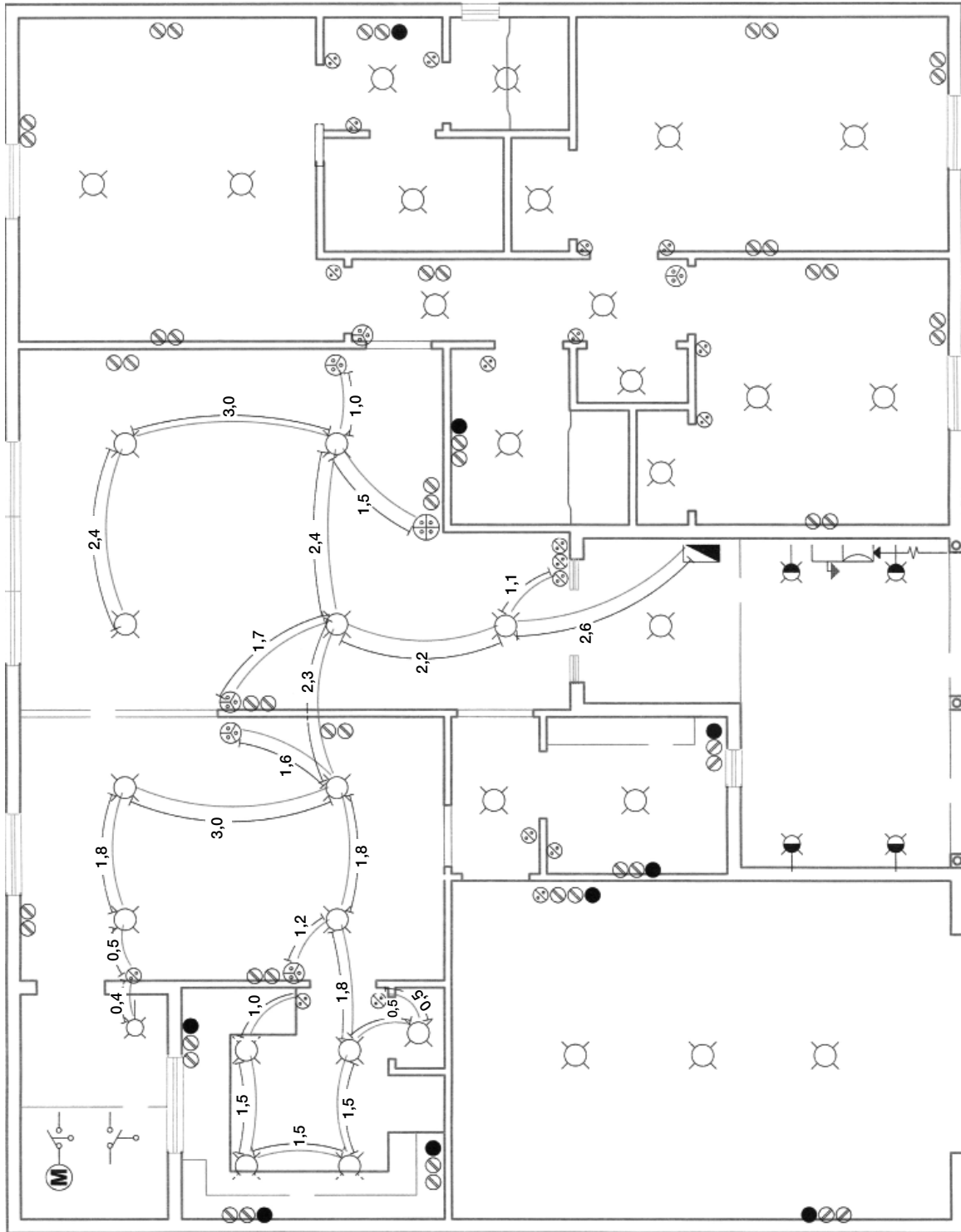
Figura 4.20. Alambrado circuito 4. Dimensiones.
