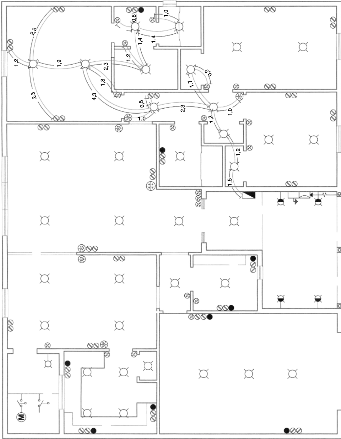
Figura 4.19. Alambrado circuito 3. Dimensiones.
